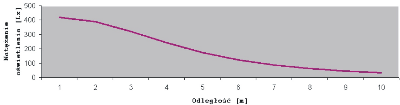
Nateżenie oświetlenia wokół lampy HTI 1000
